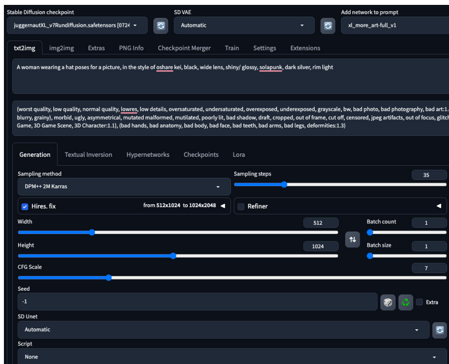
Stable Diffusion
